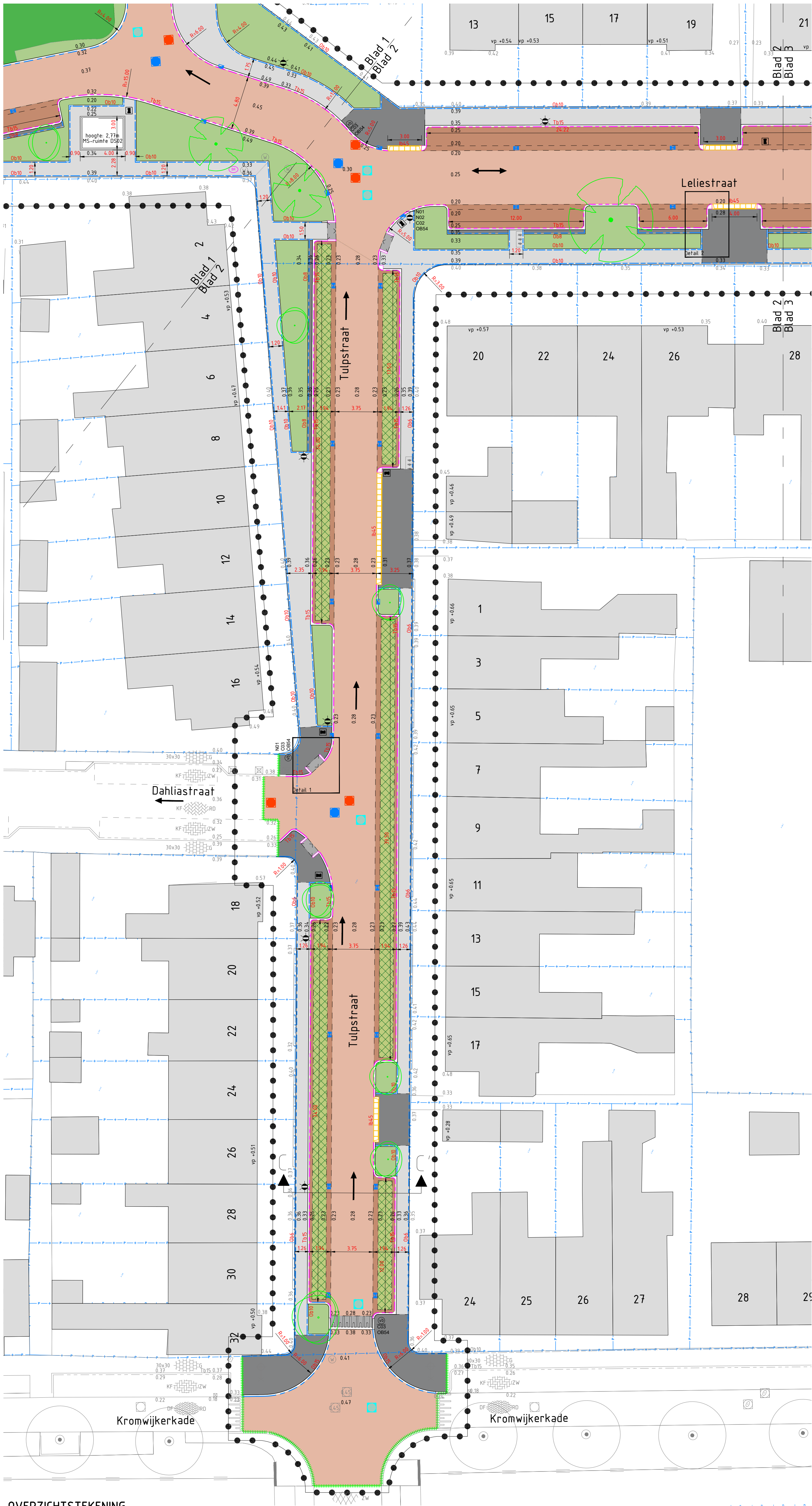
OVERZICHTSTEKENING SCHAA 1:200
