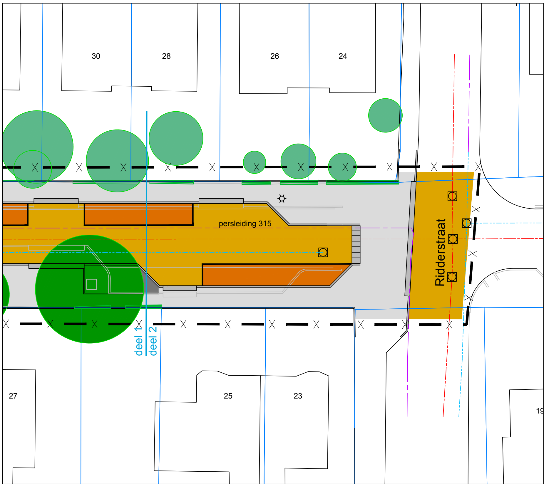
NIEUWE SITUATIE SCHAAL 1:200
