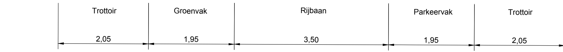
PROFIEL 2 SCHAAL 1:50
