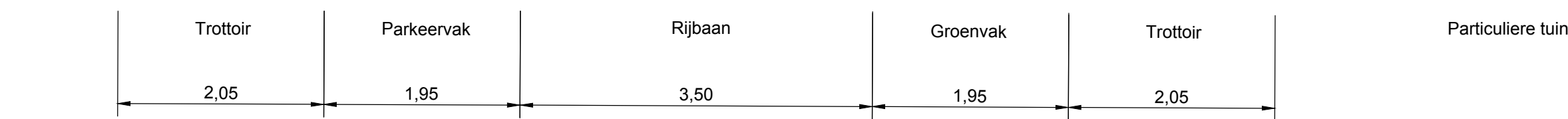
PROFIEL 1 SCHAAL 1:50
