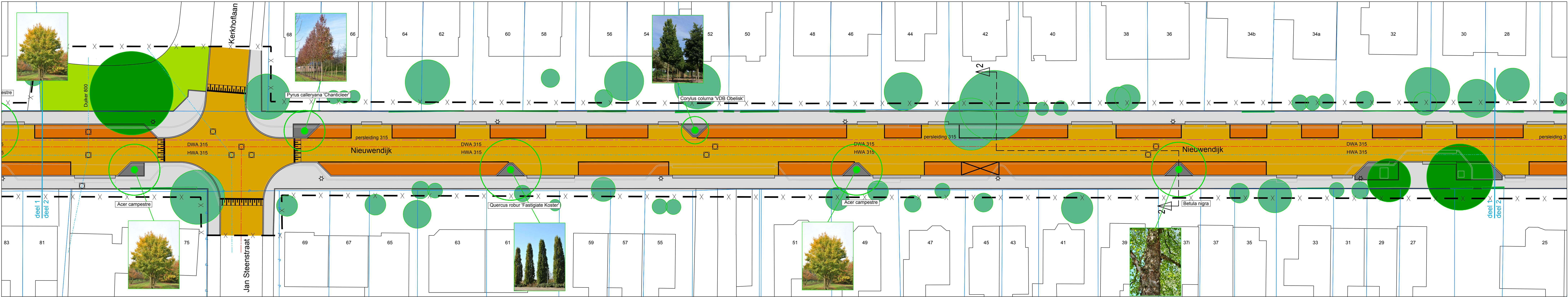
NIEUWE SITUATIE SCHAAL 1:200
